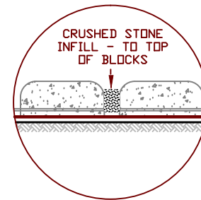
OPTIONAL STONE INFILL
